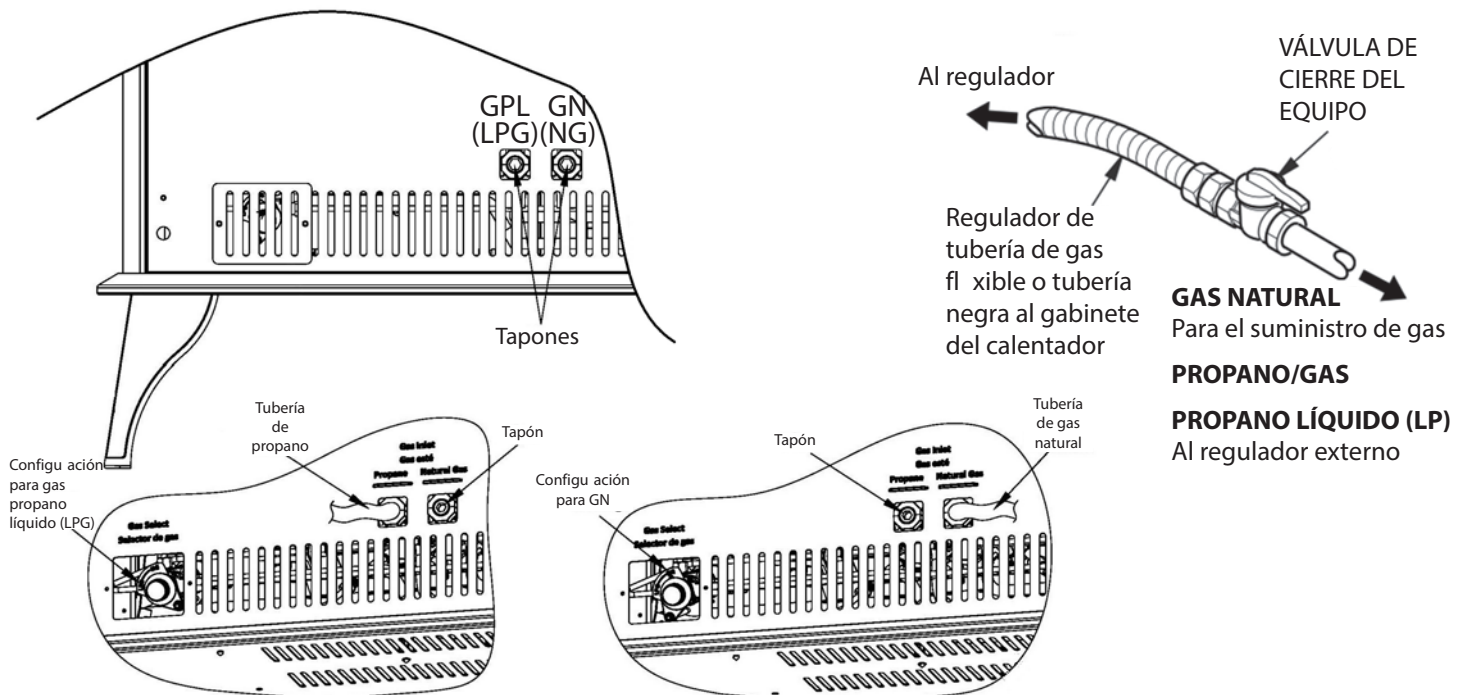
Fig. 16—Entrada de gas al regulador
